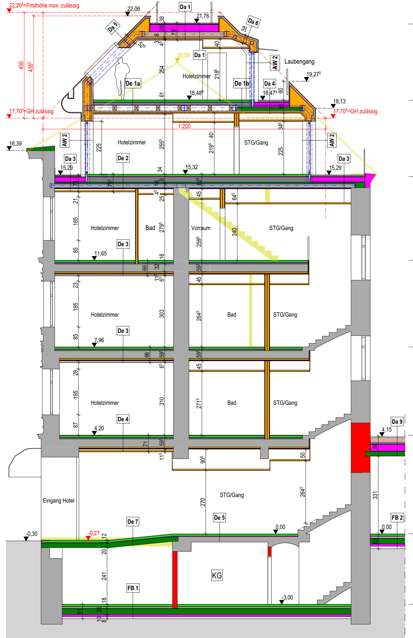
Schnitt S4
